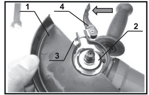
1. Protector de la rueda 2. Caja de rodamientos 3. Tornillo 4. Palanca
