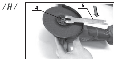
1. Flange interior 2. Protecção das rodas 3. Roda 4. Porca de segurança 5. chave de porca de segurança
